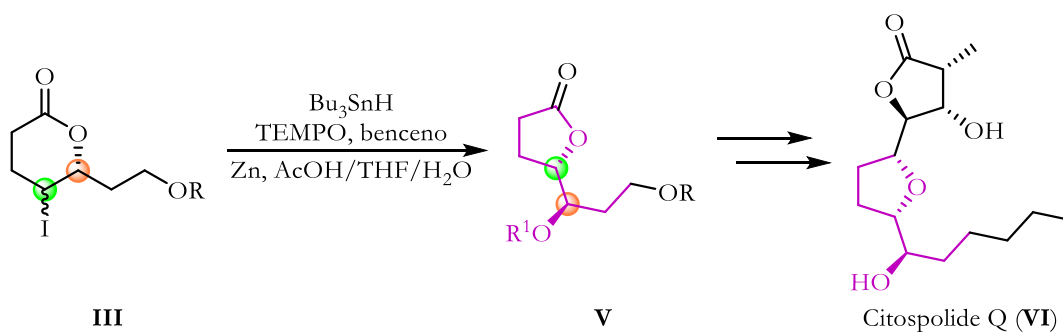
Esquema II. Propuesta sintética para el citospolide Q.
