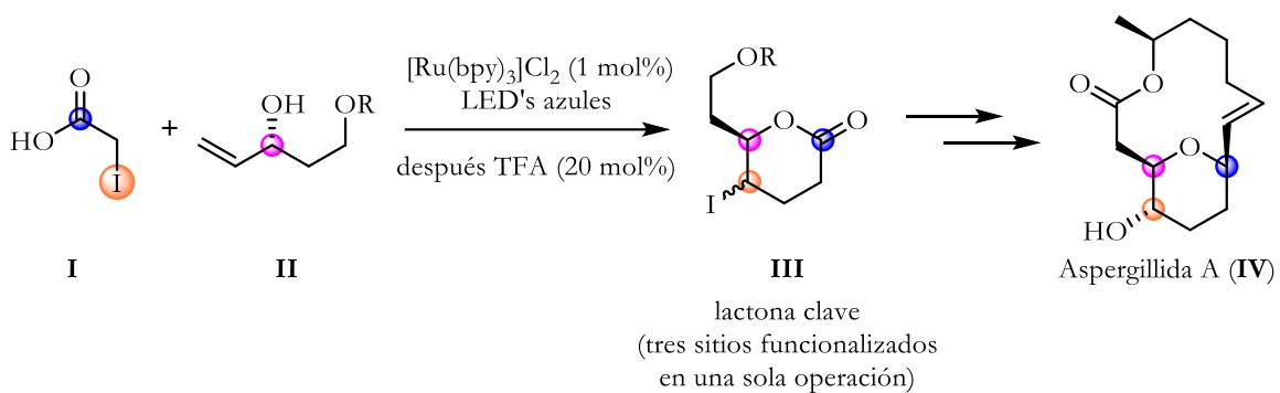
Esquema I. Síntesis total estereoselectiva de la aspergillida A.
