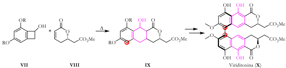
Esquema III. Aproximación sintética a la viriditoxina.
