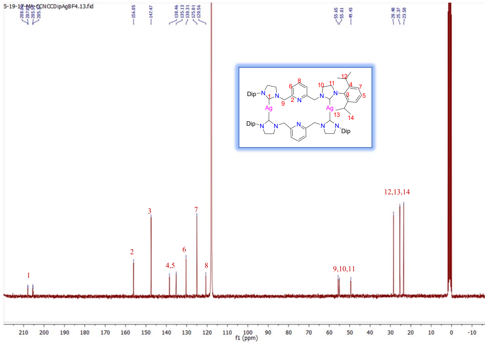
Figura 18. Espectro de ^{13}C\{^1H\} RMN del compuesto [Ag][L^1-dip][BF_4] en CD_3CN
