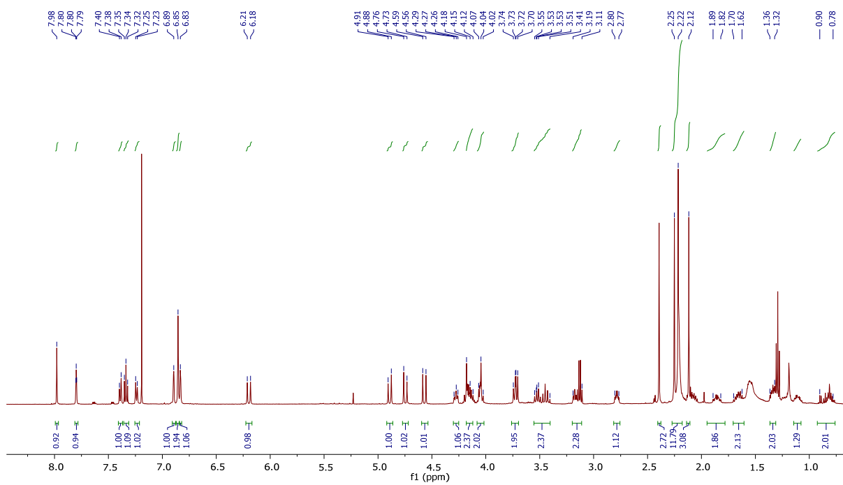
Figura S41. El espectro 1 H NMR del compuesto [Ir][L 2 -mes][Cl][PF 6 ].
