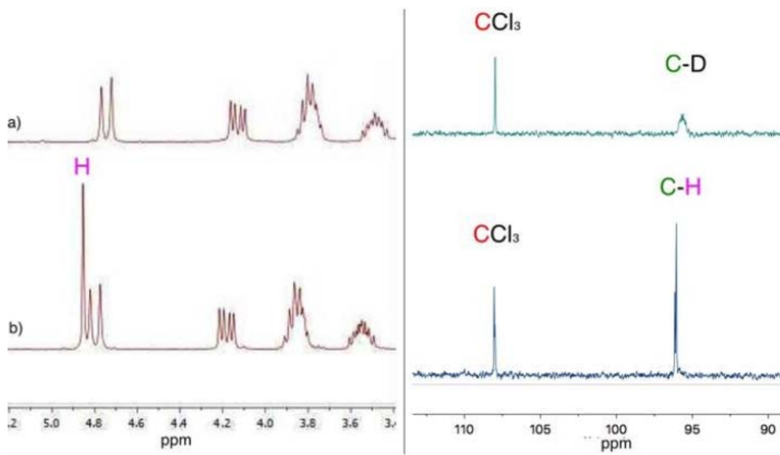
Figura 36. Vista ampliada de la ^1\text{H} RMN (izquierda) y ^{13}\text{C} (derecha) de [L^2\text{-dip}][\text{CCl}_3]\text{-d}_2 (a) y [L^2\text{-dip}][\text{CCl}_3] (b), que muestran la inclusión de deuterio en la molécula
