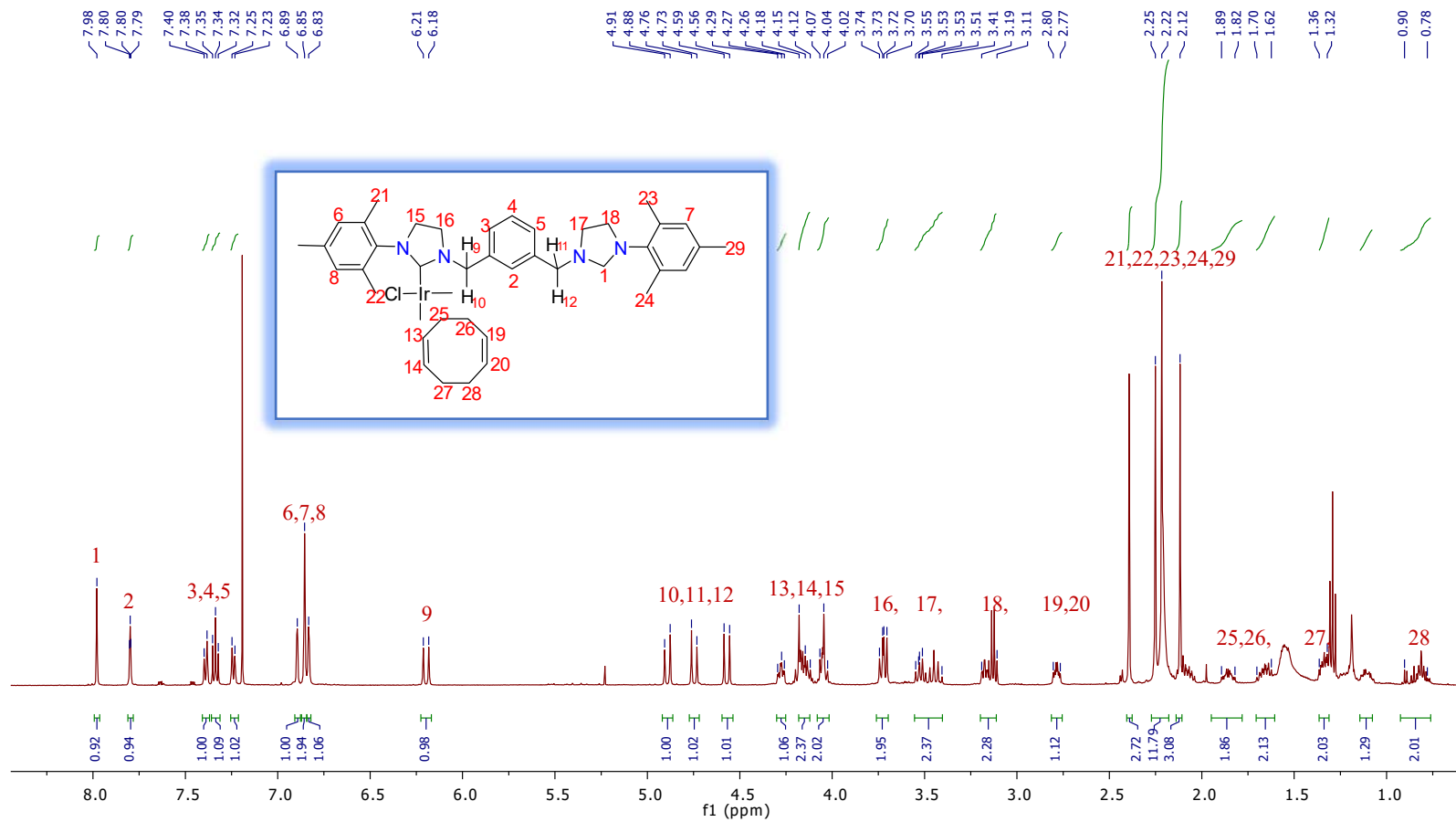
Figura 34. Espectro de ^1\text{H-NMR} del compuesto [\text{Ir}][\text{L}^2\text{-mes}][\text{Cl}][\text{PF}_6] en \text{CD}_3\text{CN}
