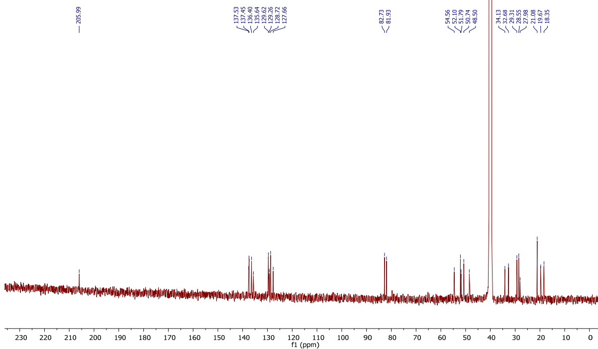
Figura S40. El espectro ^{13}\text{C} NMR del complejo diiridio [\text{Ir}_2][\text{L}^2\text{-mes}][\text{Cl}_2] .
