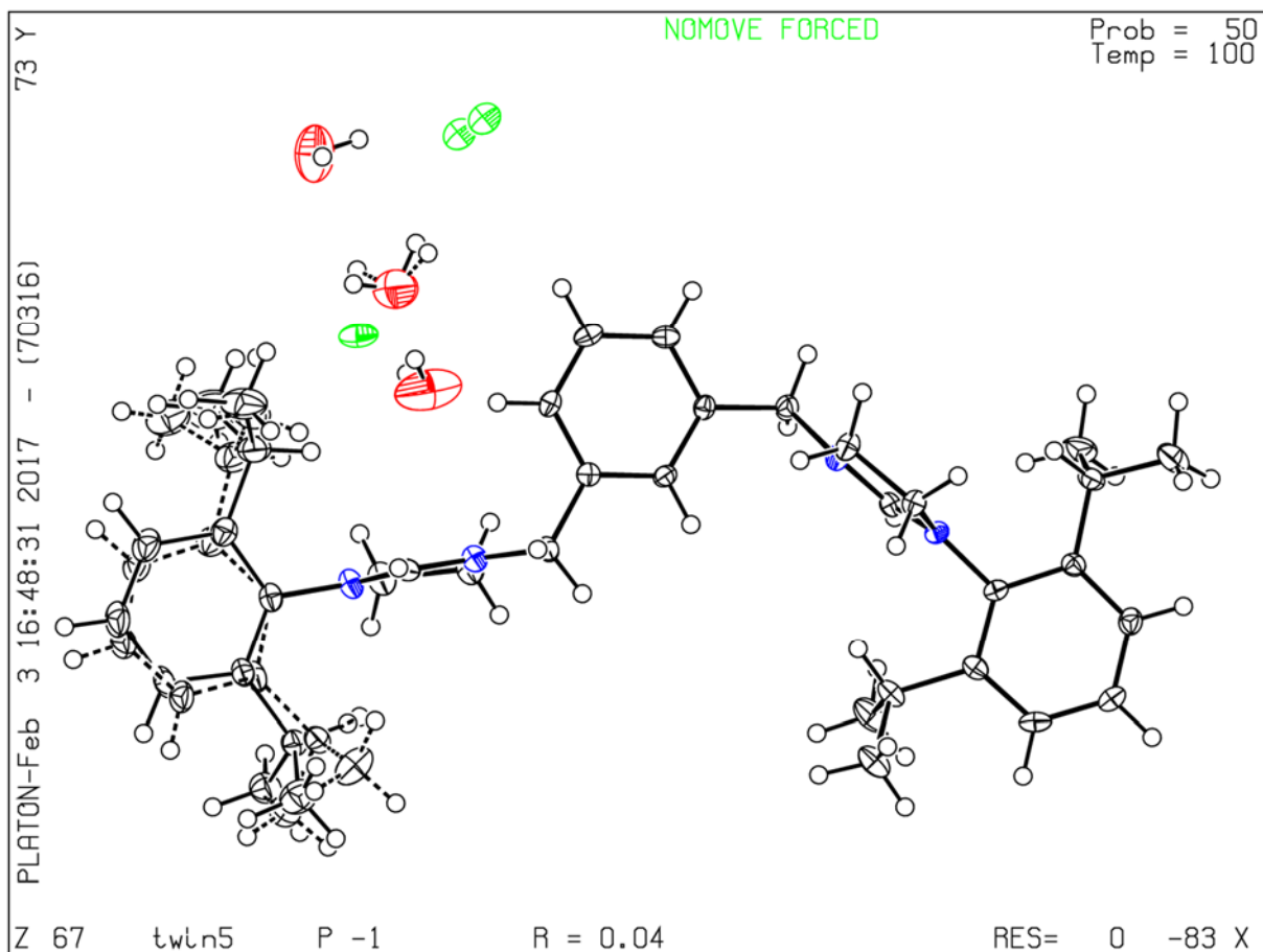
Figure S49. Estructura cristalina de rayos X de [L^2\text{-dip}][\text{Br}] .
