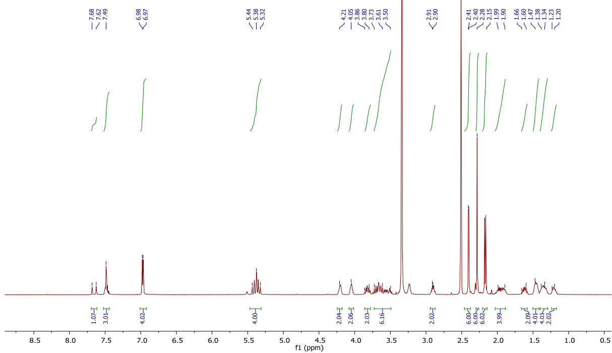
Figura S39. El espectro 1 H NMR del compuesto [Ir 2 ][L 2 -mes][Cl 2 ].
