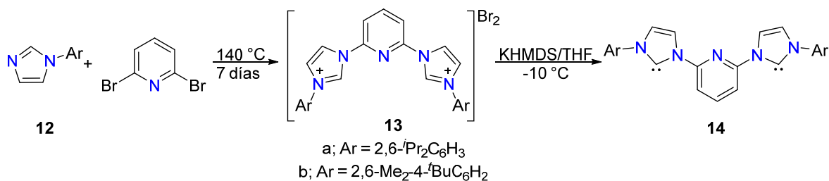
Esquema 5. Síntesis de ligantes pinza simétricos C^{NHC}NC^{NHC}
