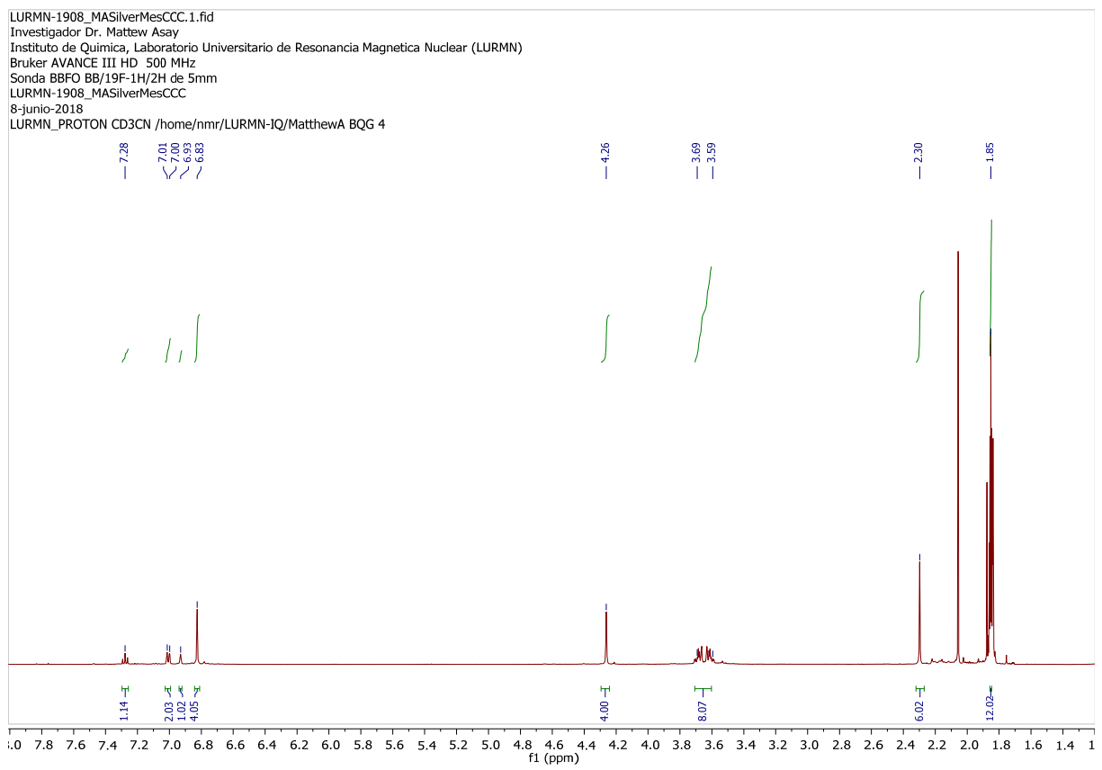
Figura S27. El espectro de 1 H NMR del compuesto [Ag][L 2 -mes][PF 6 ].
