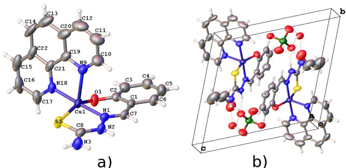
Figura 72: Estructura cristalina del compuesto 7a: a) complejo metálico y b) celda unitaria (elipsoides térmicas al 50 % de probabilidad).
