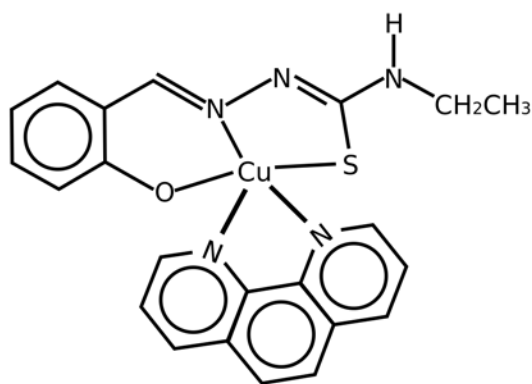
Figura 55: Fenantrolina(salicilden-3-etiltiosemicarbazonato)cobre(II). Cu(salTSC - Et)(fen) 9 .
