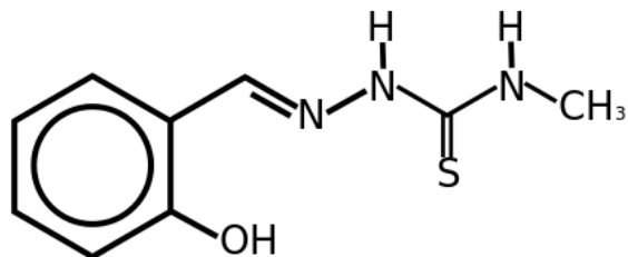
Figura 46: Salicilaldehído-3-metiltiosemicarbazona, salTSC – Met 2 .
