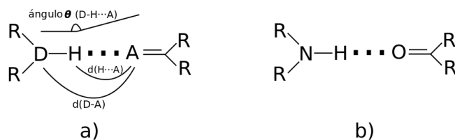
Figura 8: a) Representación de un enlace de hidrógeno y parámetros geométricos que lo caracterizan, b) Enlace de hidrógeno entre una amina secundaria y un grupo carbonilo (adaptada de J. W. Steed; D. R. Turner. John Wiley and Sons, Ltd. Inglaterra, 2007) [3].
