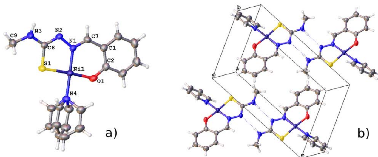
Figura 66: Ni(salTSC - Met)(py) 5 : a) unidad asimétrica y b) celda unidad.
