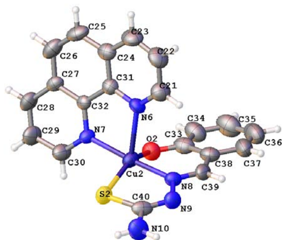
Figura 73: Complejo neutro Cu(salTSC)(fen) [42] (elipsoides térmicas al 50 % de probabilidad).
