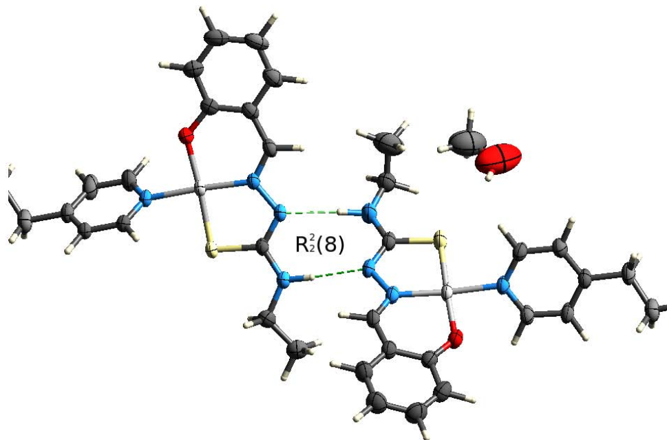
Figura 88: Síntón presente en la red cristalina de Ni_2(salTSC - Et)_2(BIS) \cdot MeOH 11 .
