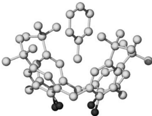
Figura 7: Estructura de rayos-x del complejo supramolecular p-terbutilcalix[4]areno-tolueno, [2].
