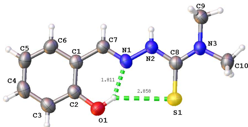
Figura 23: Salicilaldehído-3,3-dimetiltiosemicarbazona en configuración syn [36].
