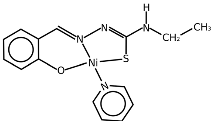
Figura 51: Piridina(salicilden - 3 - etiltiosemicarbazonato) níquel(II), Ni(salTSC - Et)(py) 6 .
