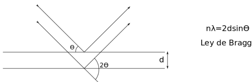
Figura 17: Representación esquemática del fenómeno de difracción de rayos X por los planos en un cristal. Los parámetros descritos están relacionados mediante la Ley de Bragg.
