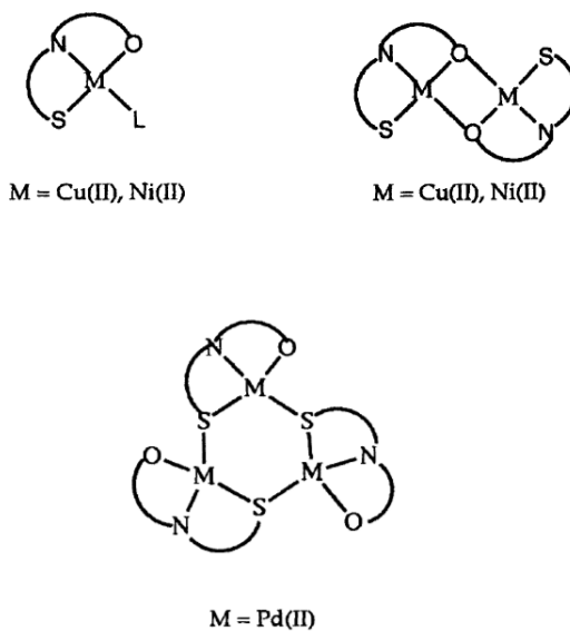
Figura 29: Modos de coordinación de tiosemicarbazonas derivadas del salicilaldehído y 2-hidroxiacetofenona [40].
