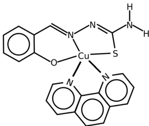
Figura 53: Fenantrolina(salicilden-tiosemicarbazonato)cobre(II), Cu(salTSC)(fen) 7 .
