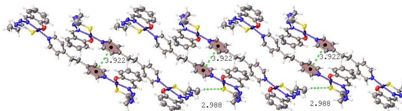
Figura 92: Complejos dinucleares de 11 en planos adyacentes que se unen gracias a enlaces de hidrógeno débiles C - H \cdots S . Las interacciones tipo \pi mostradas corresponden a las descritas en la Figura 90.
