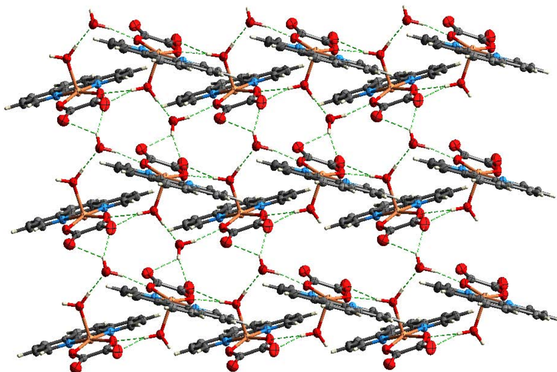
Figura 98: Planos formados en el compuesto 12 gracias a los enlaces de hidrógeno propagados en las direcciones 1 y 2 .
