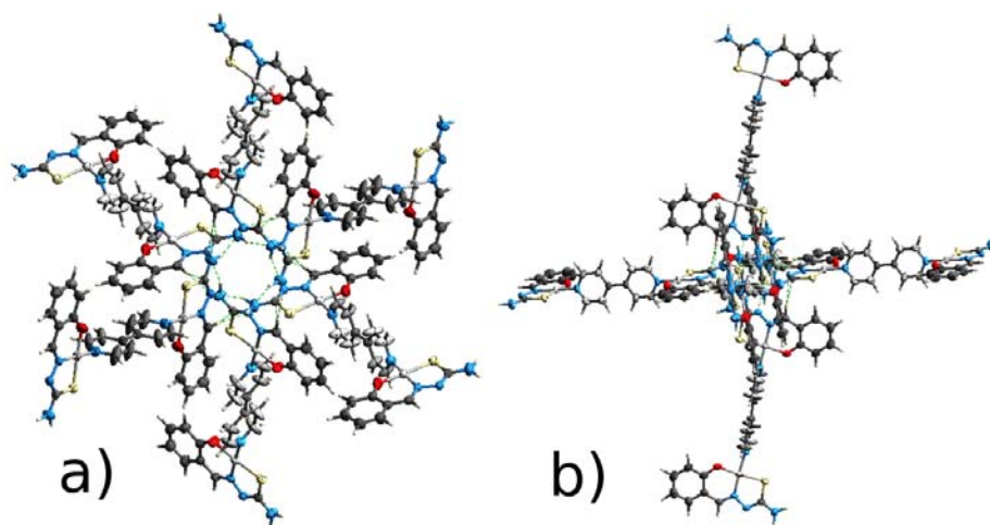
Figura 80: Vistas del arreglo hexagonal en la red cristalina de Ni_2(salTSC)_2(bipy) 10 formado a través de enlaces de hidrógeno.
