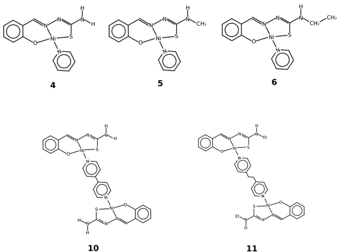
Figura 113: Complejos de níquel(II) derivados de salicilaldehído-tiosemicarbazonas.
