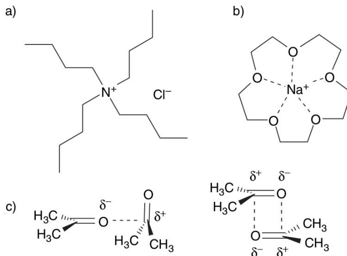
Figura 3: Ejemplos de interacciones electrostáticas: a) ión-ión en el cloruro de tetrabutilamonio; b) ión-dipolo en el complejo de sodio con el 15-corona-5; c) dipolo-dipolo en la acetona [3].
