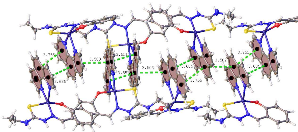
Figura 108: Cadenas de complejos metálicos formadas por interacciones aromáticas (OFF) en el cristal entre complejos [Cu(salTSC - Et)(fen)]^+ en 14 .
