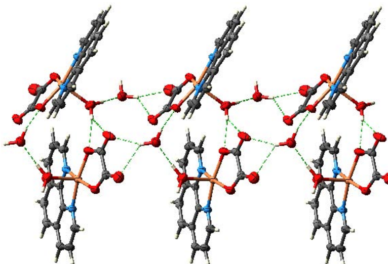
Figura 97: Enlaces de hidrógeno en el compuesto 12 , formados a través de los ligantes acua y oxalato (dirección 2 ).
