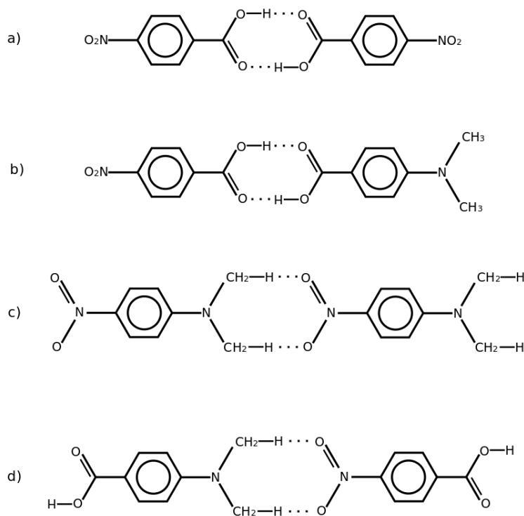
Figura 14: a) homosintón homodimérico, b) homosintón heterodimérico, c) heterosintón homodimérico y d) heterosintón heterodimérico [8].
