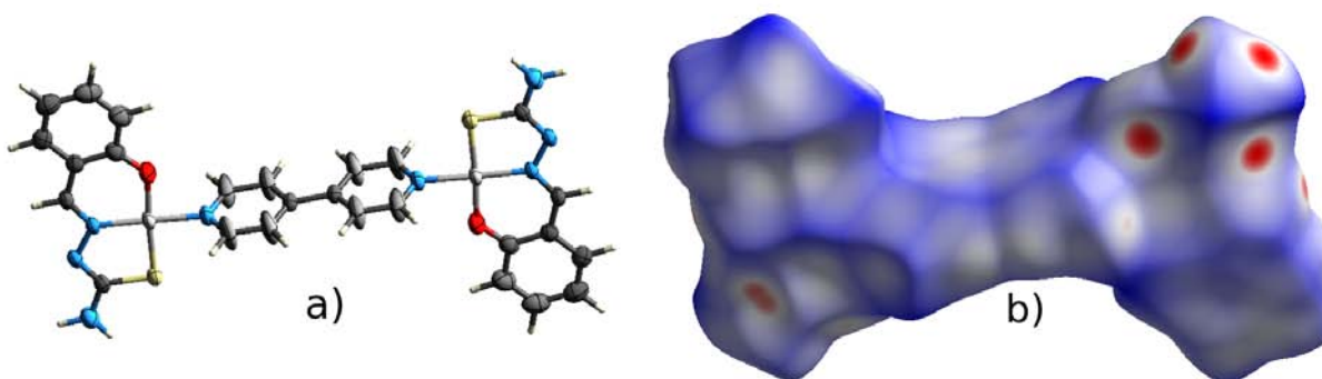
Figura 79: Superficie de Hirshfeld para el compuesto Ni_2(salTSC)_2(bipy) 10 mapeada con d_{norm} .
