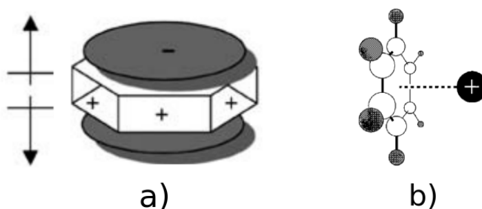
Figura 4: a) momento cuadrupolar del benceno, b) interacción de un catión genérico con la cara de un anillo aromático. (Adaptado de “the cation- \pi Interaction”. J. C. Ma; D. A. Dougherty. Chem. Rev. 1997 [6]. y de “Supramolecular Chemistry”. J. W. Steed; J. L. Atwood. John Wiley and Sons, Ltd. Inglaterra, 2000.) [2].
