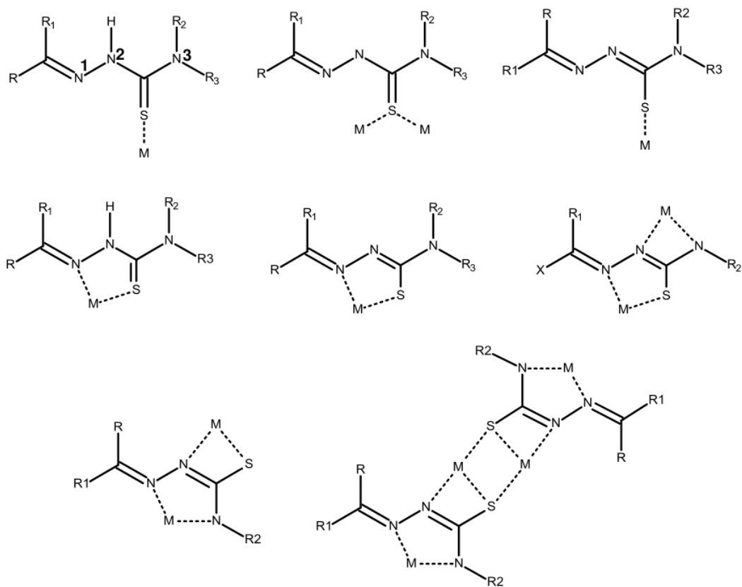
Figura 28: Modos de coordinación de tiosemicarbazonas [5].
