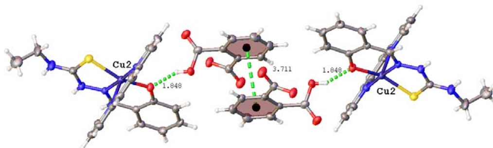
Figura 111: Enlaces de hidrógeno entre el oxígeno del fragmento tiosemicarbazona y el anión ftalato que resulta en la asociación de cadenas vecinas.
