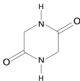
Figura 18: Estructura de la 2,5-diketopiperazina.
