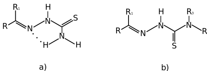
Figura 21: Configuraciones más comunes en tiosemicarbazonas: a) anti ( E ) y b) syn ( Z ).
