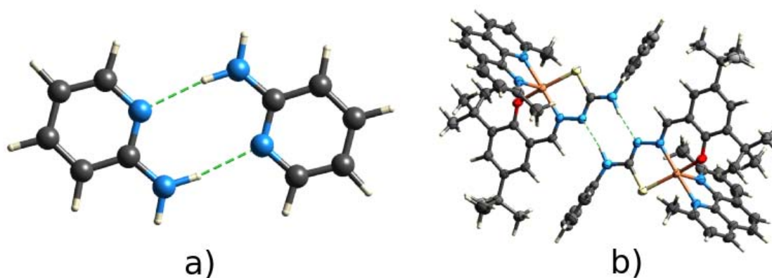
Figura 43: Enlaces de hidrógeno complementarios en las moléculas de: a) 2-aminopiridina [57] y b) Cu(salTSC)(fen) ; donde salTSC=3,5 -di- t -butilsalicilaldehído-3-feniltiosemicarbazona y fen=2,9 -dimetil-1,10-fenantrolina [42].
