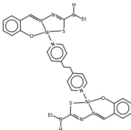
Figura 58: bis[salicilden-3-etiltiosemicarbazonato]níquel(II) 1,2-bis(4-piridil)etano. Ni_2(\text{salTSC} - \text{Et})_2(\text{BIS}) 11.
