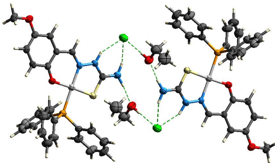
Figura 36: Complejación de aniones cloruro por el compuesto [Ni(5-MeO-HSalTSC)PPh_3]^+ [35].
