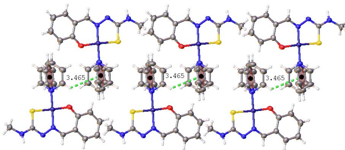
Figura 70: Interacciones tipo C - H \cdots \pi en el compuesto Ni(salTSC - Met)(py) 5 .
