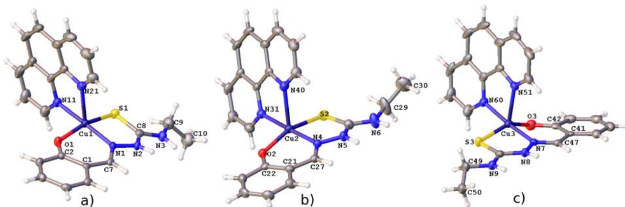
Figura 107: Complejos [Cu(\text{saltTSC} - Et)(\text{fen})]^+ de la unidad asimétrica en 14 con conformaciones diferentes: a) Cu1 , b) Cu2 y c) Cu3 .
