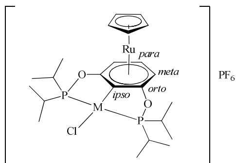
Figura 4. Nomenclatura usada para la asignación de señales en RMN.
