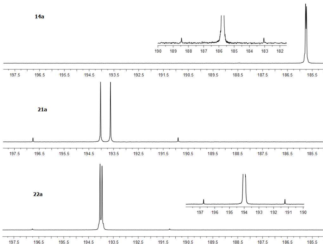
Figura 5. RMN- ^{31}\text{P}\{\text{H}\} de 14a (en \text{CDCl}_3 ), 21a y 22a (en \text{CD}_2\text{Cl}_2 ) a temperatura ambiente.
