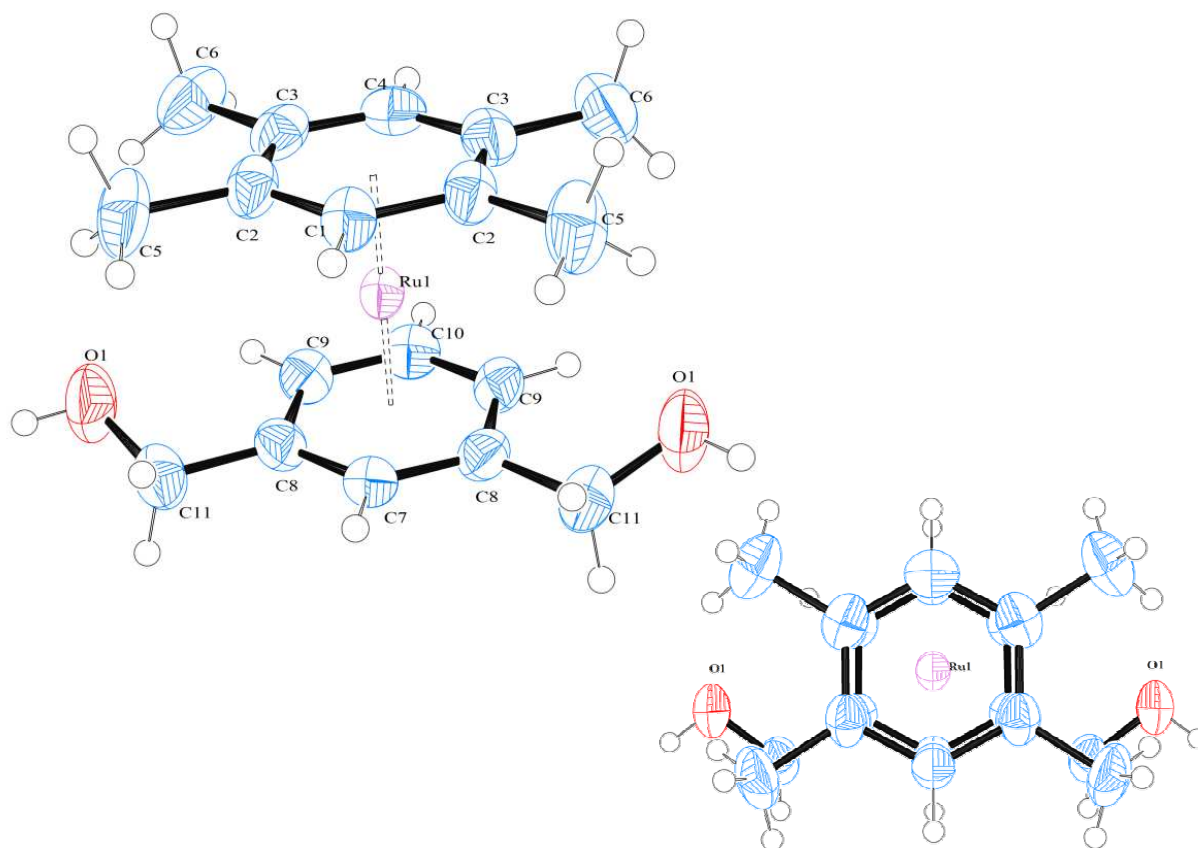
Figura 16. Vistas ORTEP del complejo [\mathbf{11}](\text{PF}_6)_2 . Los elipsoides térmicos están dibujados a un nivel del 50% de probabilidad. El anión es omitido para mayor claridad.
