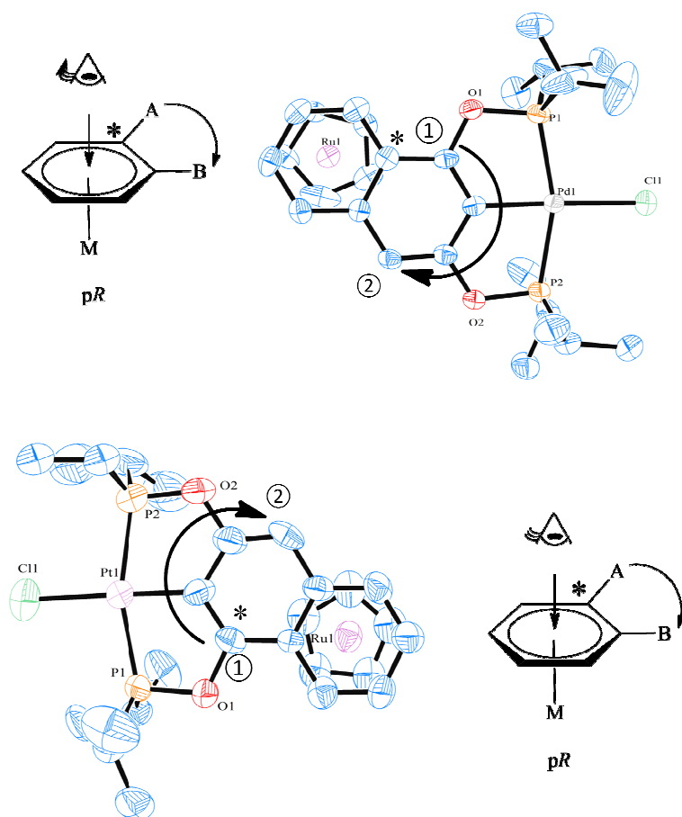
Figura 10. Asignación de las configuraciones absolutas para crisales-26b (arriba) y crisales-26c (abajo).
