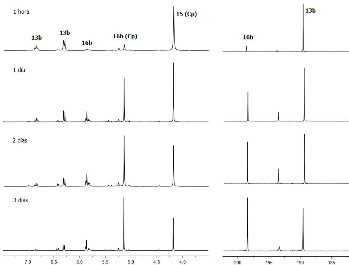
Figura 1. Ampliaciones de los espectros de RMN- ^1\text{H} (izquierda) y RMN- ^{31}\text{P}\{^1\text{H}\} (derecha) en \text{CD}_2\text{Cl}_2 a diferentes tiempos (1 hora, 1 día, 2 días, 3 días respectivamente) para la formación de 16b . La reacción se realizó en un tubo de RMN, sellado y sin agitación a temperatura ambiente.
