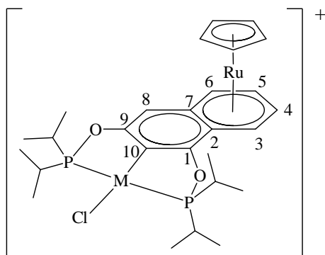
Figura 4. Numeración usada en la asignación de señales en RMN.
