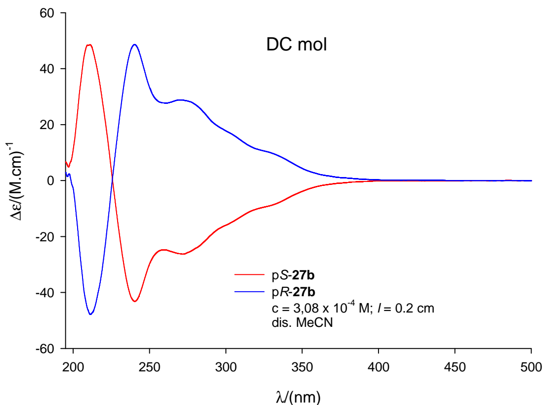
Gráfica 2. Curvas de DC para los enantiómeros de 27b .
