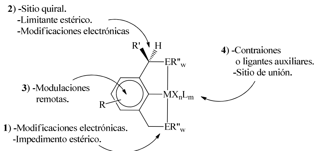
Esquema 8. Sitios de potencial modificación y sus efectos al centro metálico.
