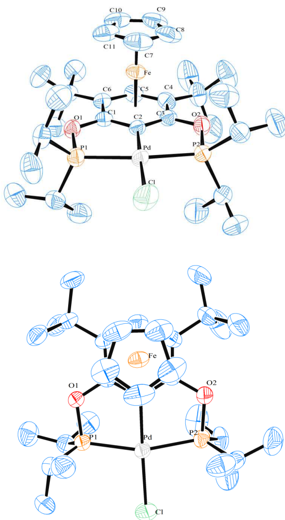
Figura 6. Vista ORTEP del complejo 19b . Los elipsoides térmicos están dibujados con un 50% de probabilidad. Los átomos de hidrógeno y el anión PF 6 - son omitidos para más claridad.
