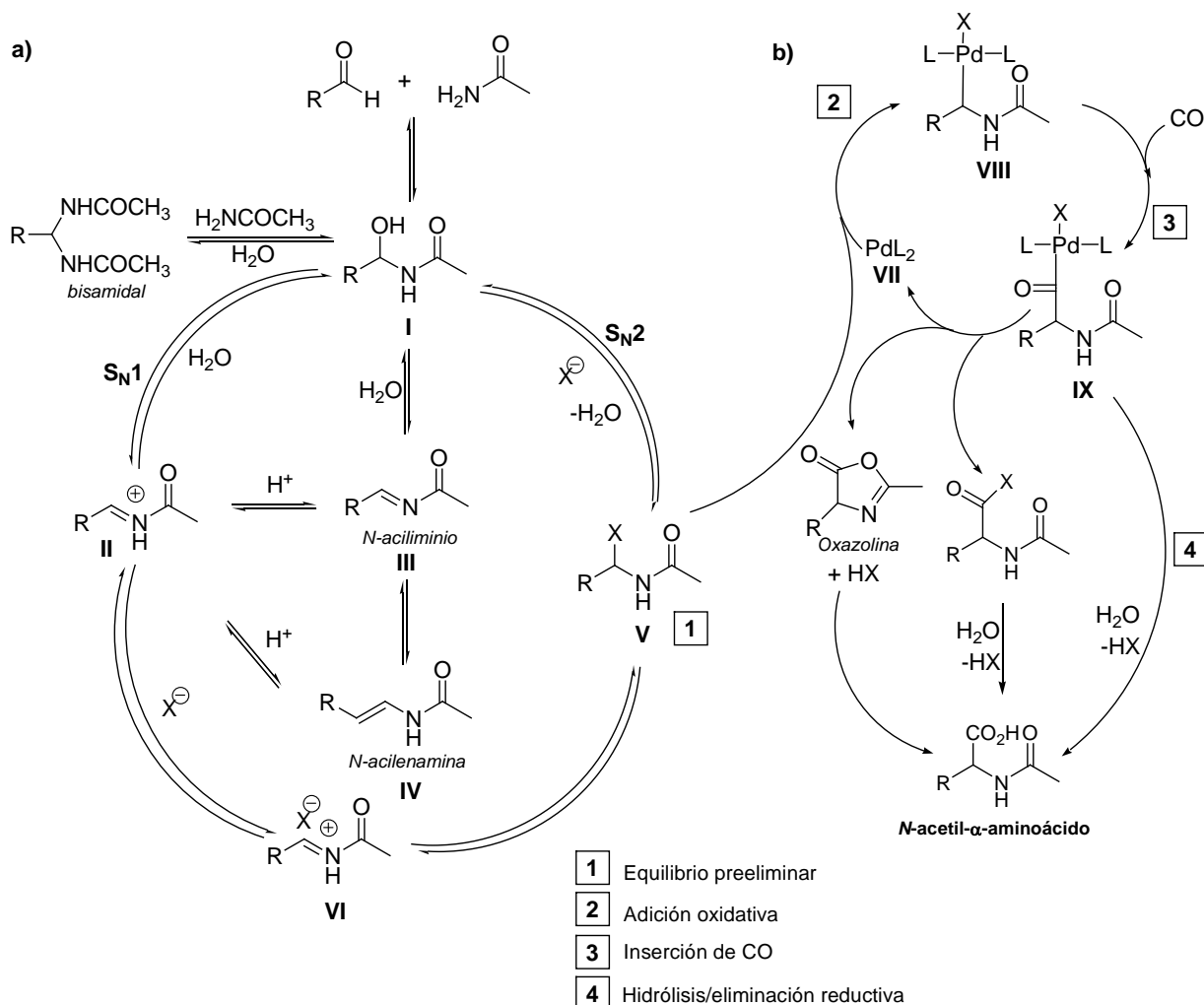
Esquema 5.3. Ciclo catalítico propuesto por Beller.
