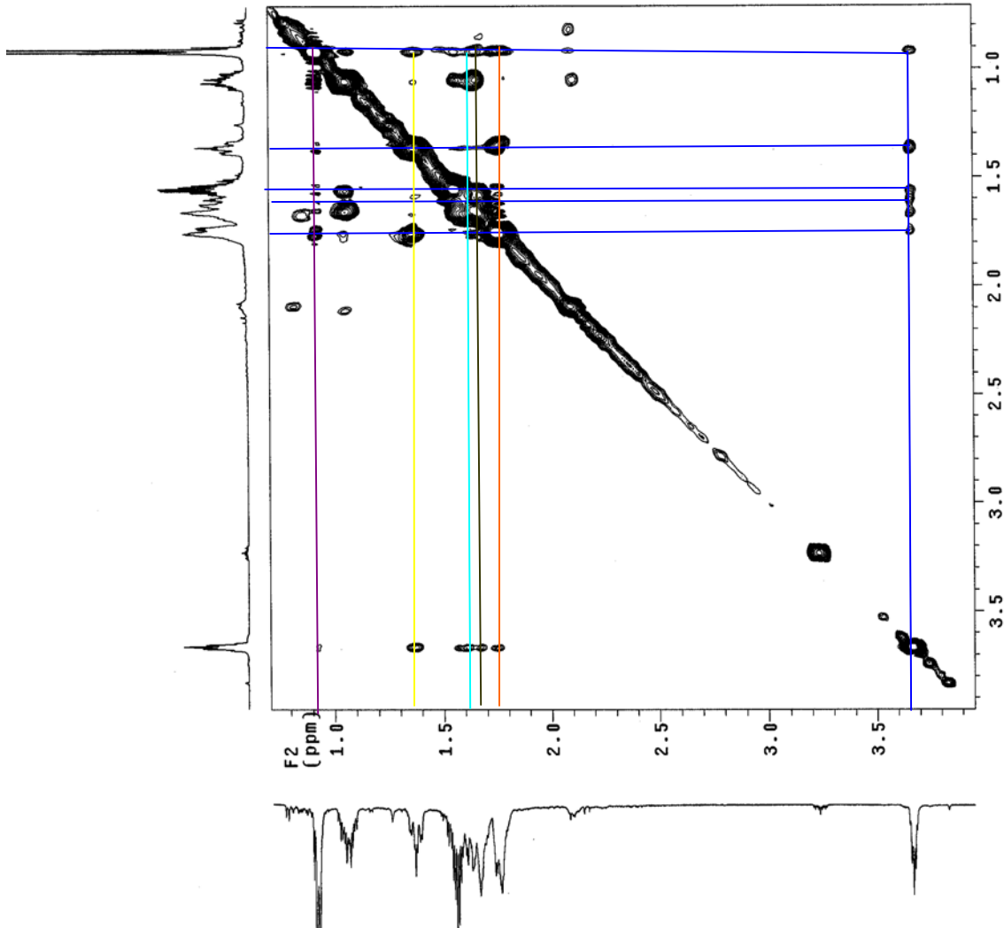
Anexo experimental D.47. Ampliación del espectro bidimensional NOESY del compuesto 13a (zona alifática).
