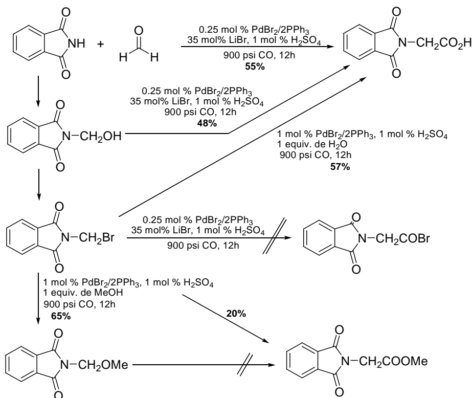
Esquema 5.4. Investigaciones mecanísticas sobre la amidocarbonilación de ftalimida con formaldehído catalizada con paladio.
