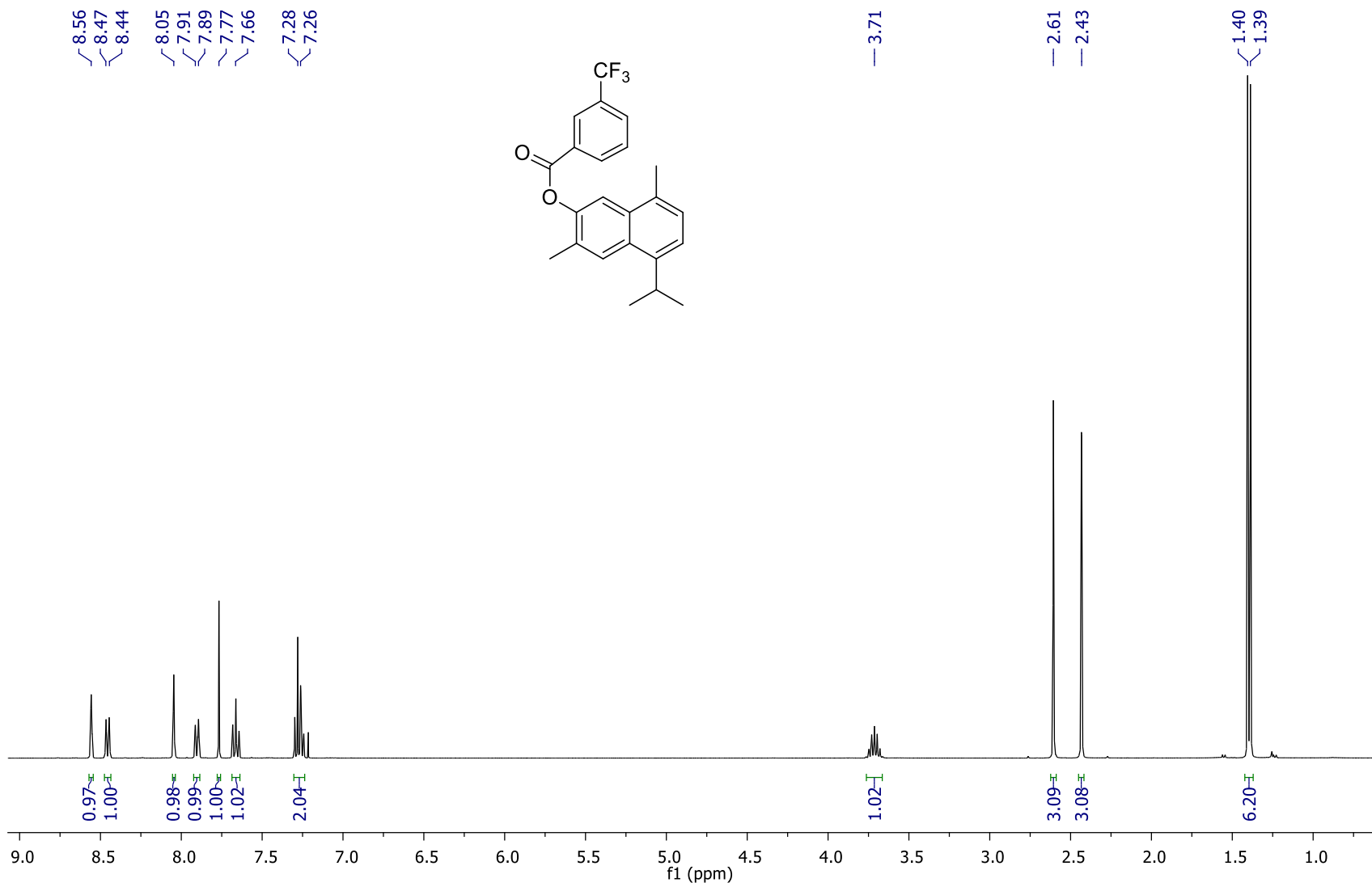
Espectro 35. RMN ^1\text{H} del compuesto 30 (400 MHz, \text{CDCl}_3 ).
