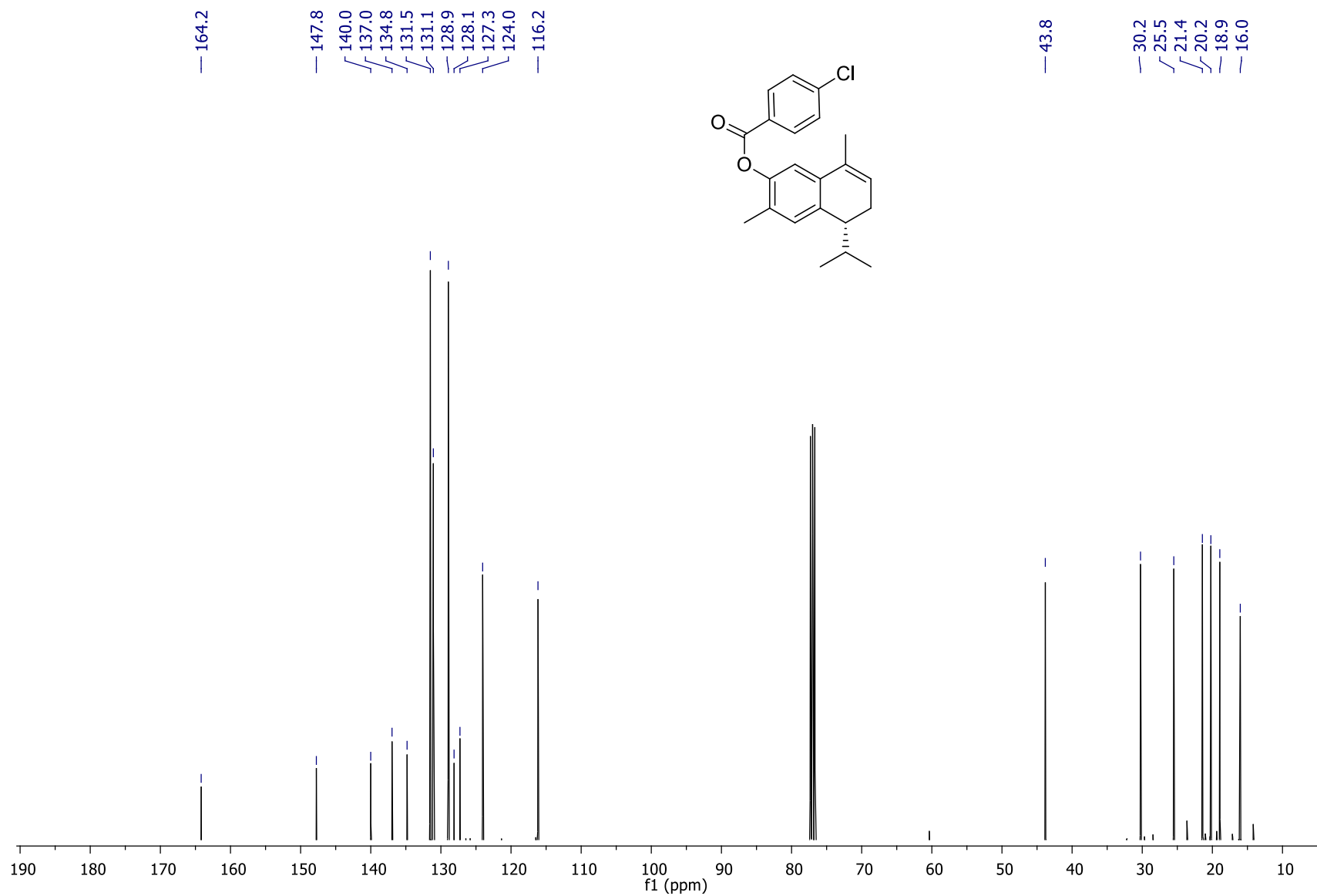
Espectro 2. RMN ^{13}\text{C} del compuesto 12 (100 MHz, \text{CDCl}_3 ).
