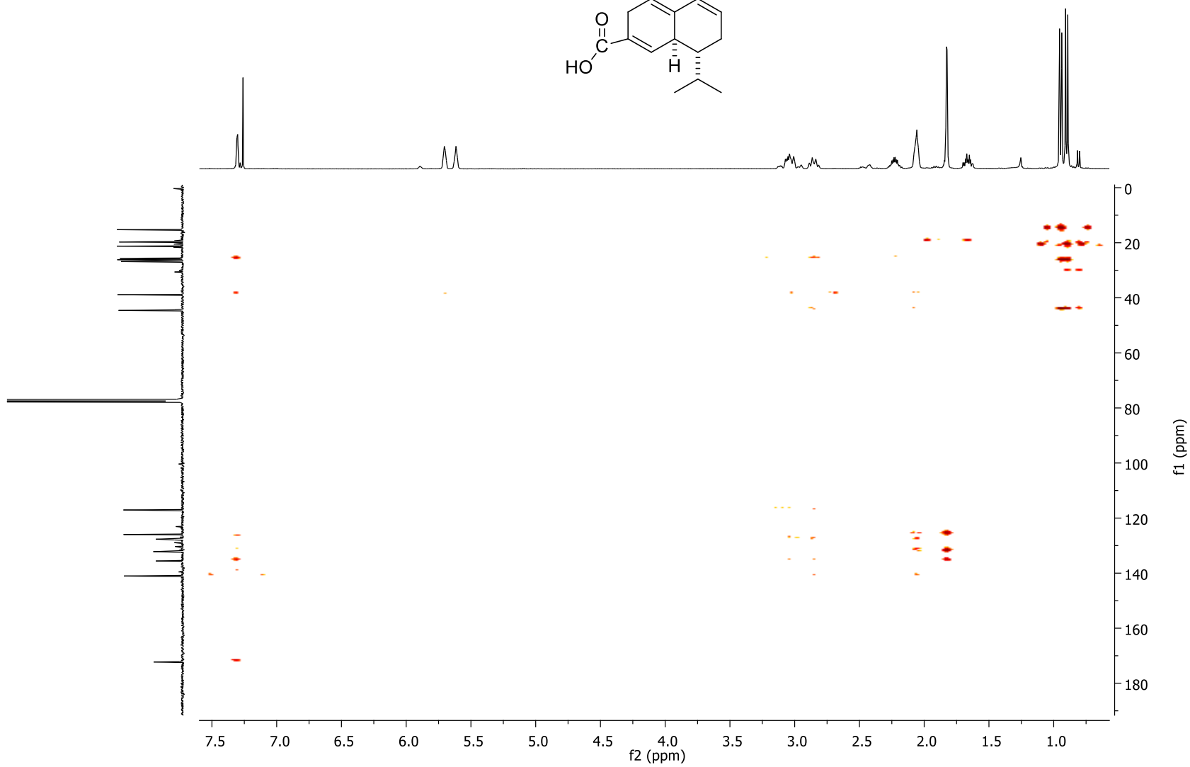
Espectro 17. HMBC del compuesto 3 (CDCl 3 ).
