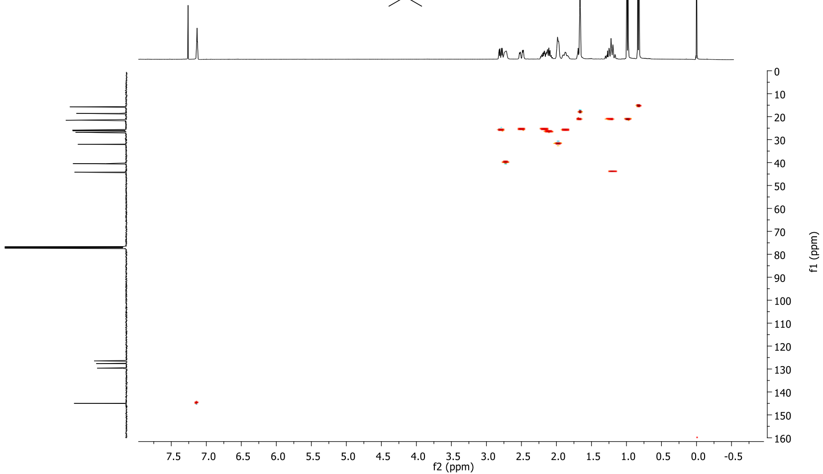
Espectro 10. HSQC del compuesto 2 ( \text{CDCl}_3 ).
