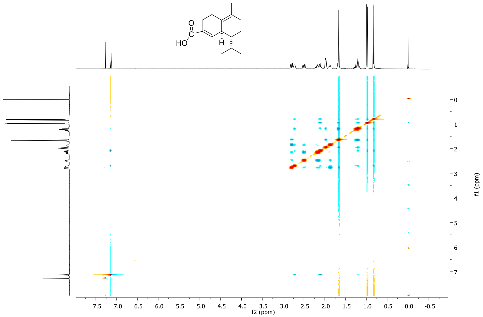
Espetro 12. NOESY del compuesto 2 ( \text{CDCl}_3 ).
