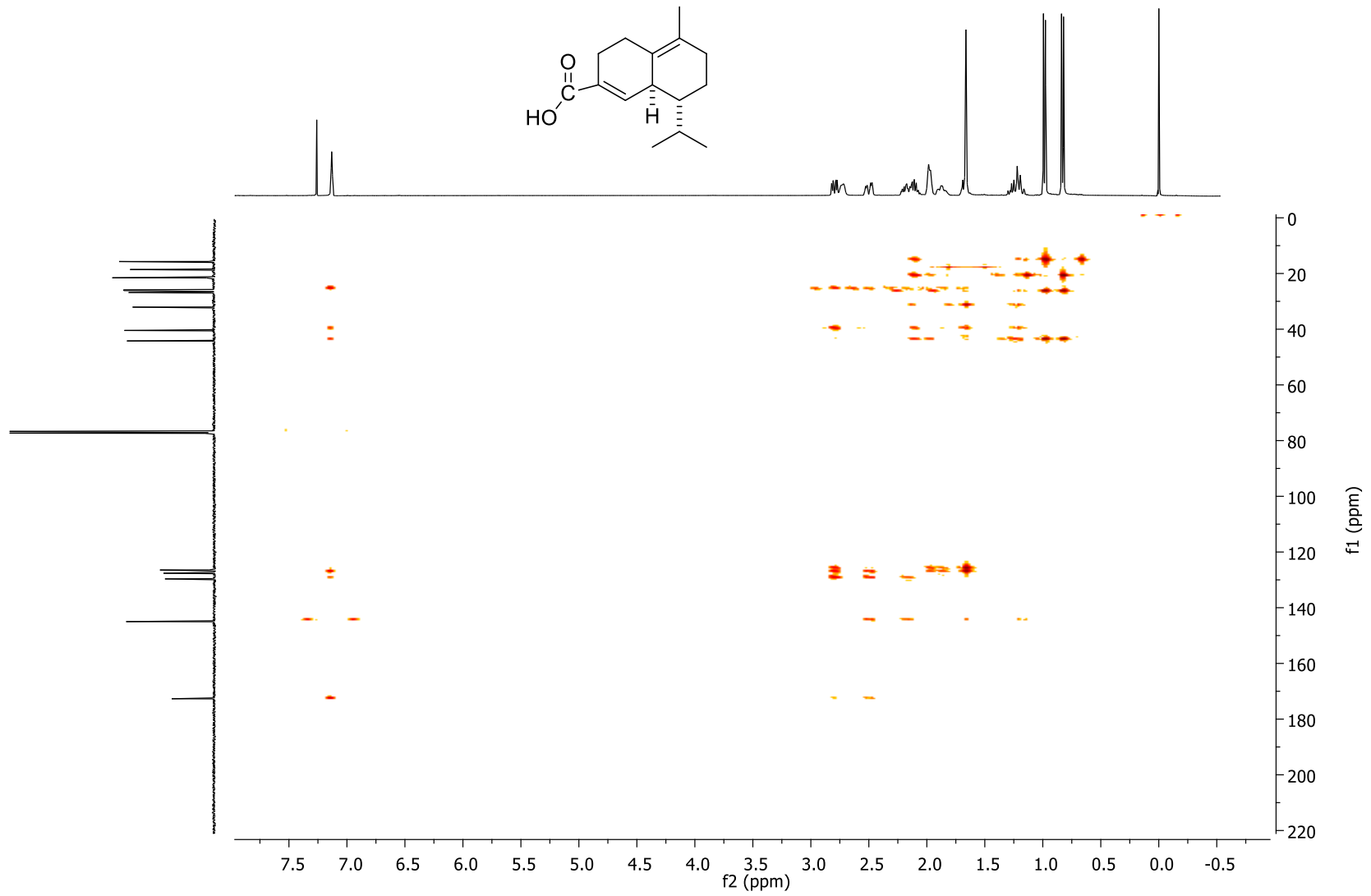
Espectro 11. HMBC del compuesto 2 (CDCl 3 ).
