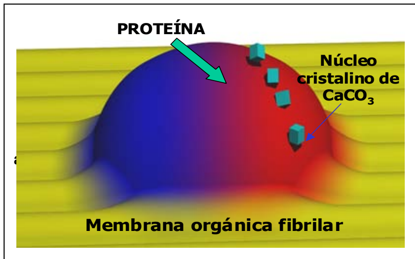
Figura 2. Representación esquemática de la nucleación del carbonato de calcio por parte de una proteína intramineral del cascarón de huevo de las aves.
