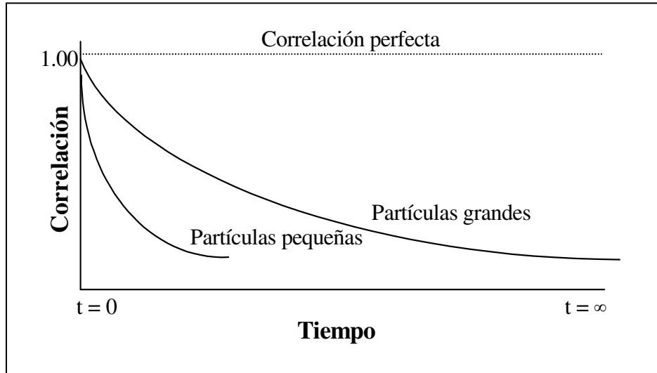
Figura 11. Función de correlación para partículas grandes y pequeñas en una medición de DLS.
