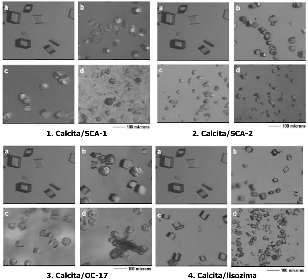
Figura 32. Cristalización de calcita en presencia de algunas proteínas intraminerales presentes en los cascarones de huevos de algunas aves. a) Imagen del control (concentración de proteína = 0.0 \mu\text{g} ), se pueden observar los cristales romboédricos perfectos de calcita. b-d) cristales de calcita crecidos bajo la presencia de 50, 100 y 200 \mu\text{g} de las proteínas respectivamente. Escala: 100 \mu\text{m} .
