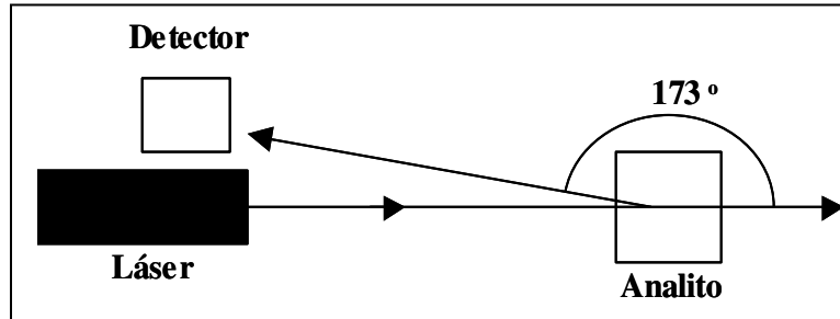
Figura 10. Representación esquemática de los componentes básicos de un equipo de DLS.
