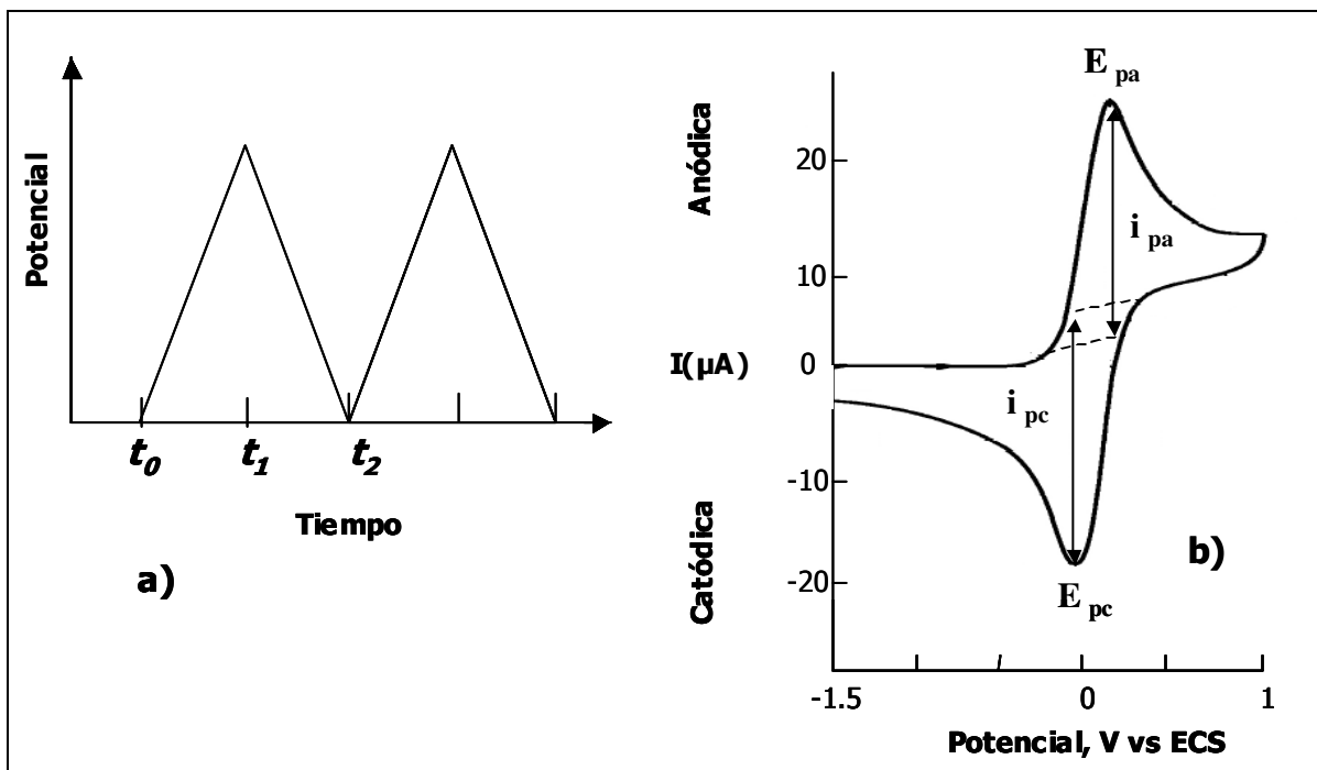
Figura 13. a) Señal de excitación en voltamperometría cíclica. b) Voltamperograma cíclico, arriba: pico anódico (oxidación), abajo: pico catódico (reducción).
